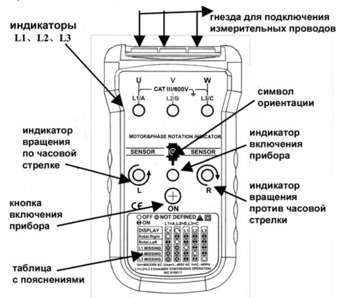
Рисунок 1. Схема прибора
