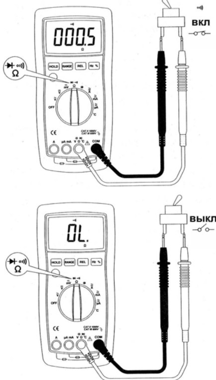
Рисунок 6. Прозвонка электрических цепей
