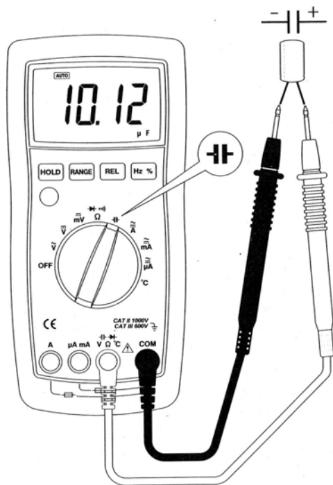
Рисунок 7. Измерение емкости
