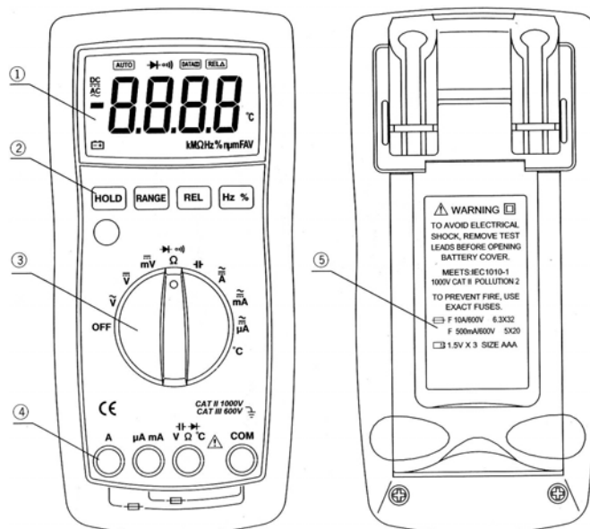
Рисунок 1. Схема мультиметра
