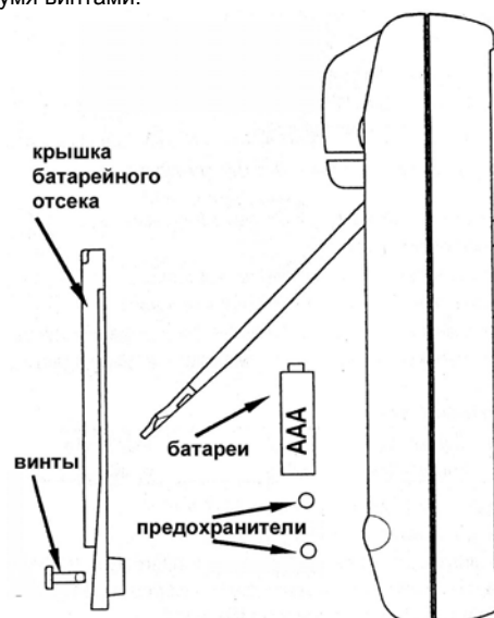
Рисунок 9. Замена батарей и предохранителей.
