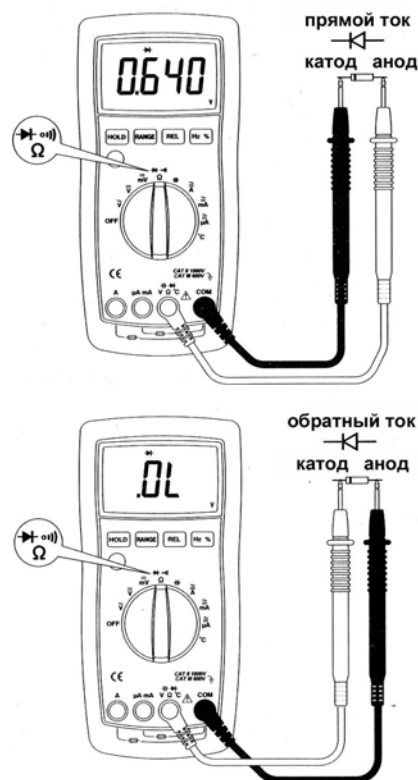
Рисунок 5. Проверка диодов
