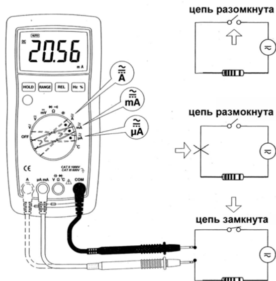
Рисунок 8. Измерение силы тока
